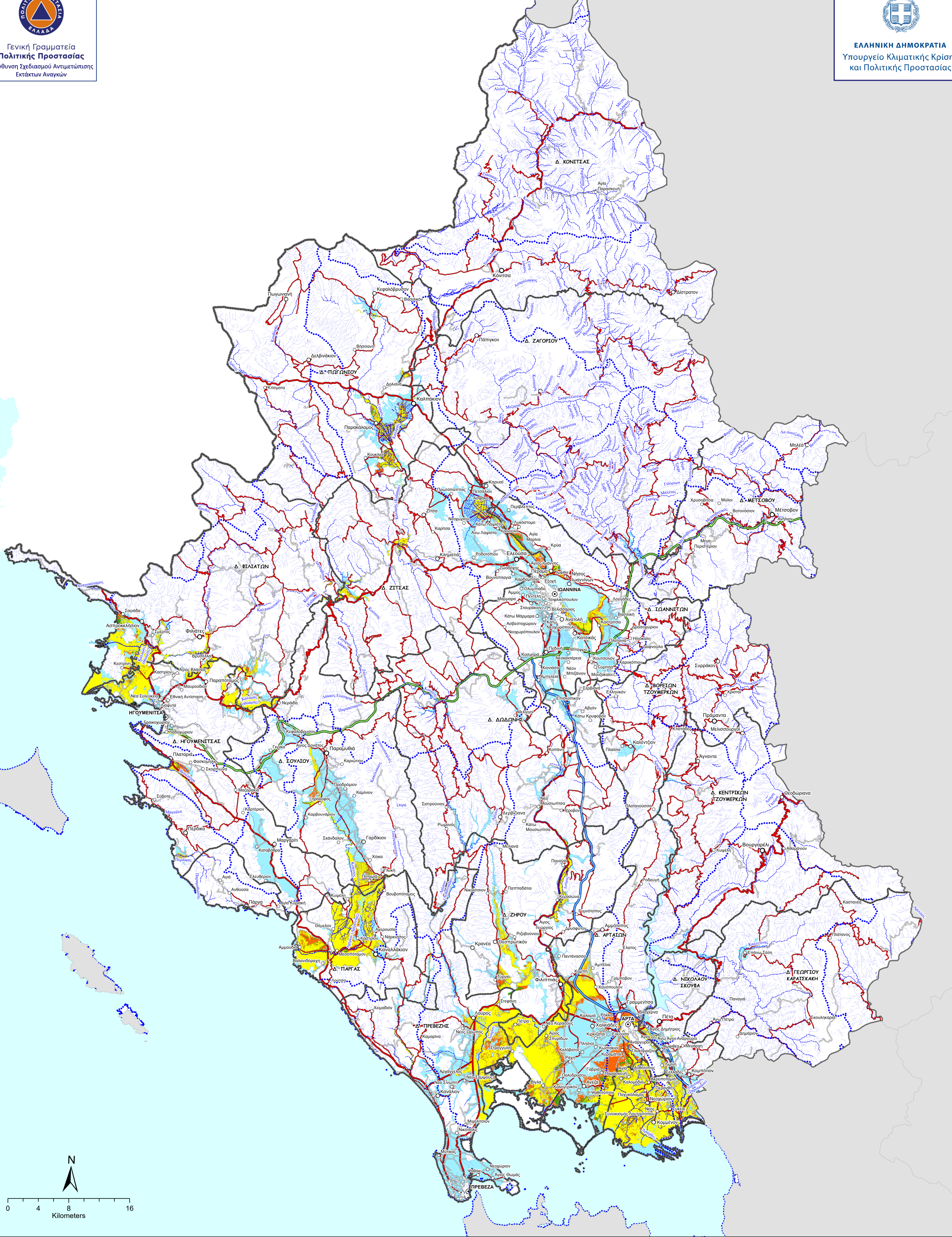
ΧΑΡΤΗΣ ΜΕ ΤΙΣ ΖΩΝΕΣ ΔΥΝΗΤΙΚΑ ΥΨΗΛΟΥ ΚΙΝΔΥΝΟΥ ΠΛΗΜΜΥΡΑΣ ΚΑΙ ΤΙΣ ΖΩΝΕΣ ΥΨΗΛΗΣ ΕΠΙΚΙΝΔΥΝΟΤΗΤΑΣ ΠΛΗΜΜΥΡΑΣ ΓΙΑ ΠΕΡΙΟΔΟ ΕΠΑΝΑΛΗΨΗΣ 50, 100 ΚΑΙ 1000 ΕΤΩΝ ΠΕΡΙΦΕΡΕΙΑ ΗΠΕΙΡΟΥ
