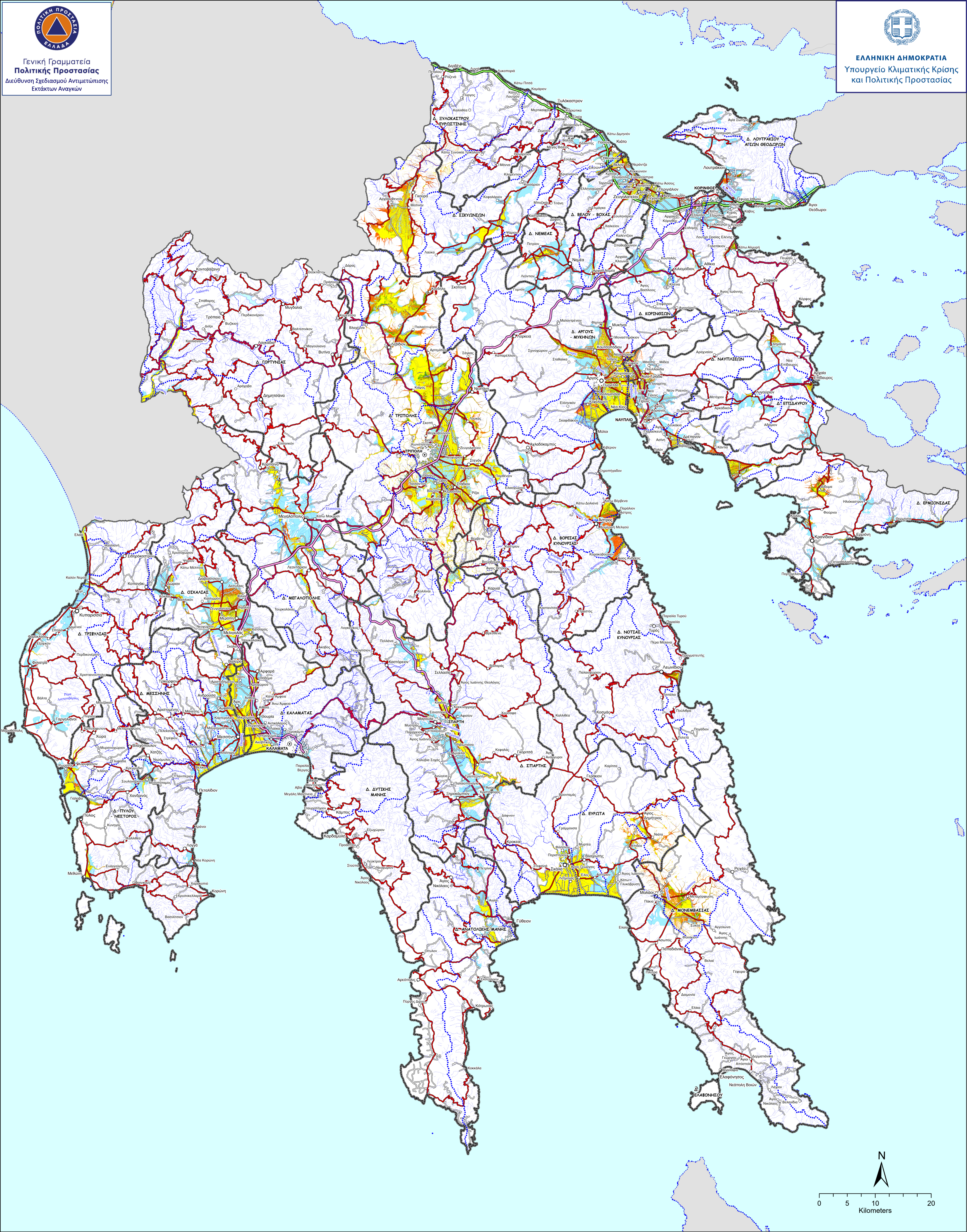
ΧΑΡΤΗΣ ΜΕ ΤΙΣ ΖΩΝΕΣ ΔΥΝΗΤΙΚΑ ΥΨΗΛΟΥ ΚΙΝΔΥΝΟΥ ΠΛΗΜΜΥΡΑΣ ΚΑΙ ΤΙΣ ΖΩΝΕΣ ΥΨΗΛΗΣ ΕΠΙΚΙΝΔΥΝΟΤΗΤΑΣ ΠΛΗΜΜΥΡΑΣ ΓΙΑ ΠΕΡΙΟΔΟ ΕΠΑΝΑΛΗΨΗΣ 50, 100 ΚΑΙ 1000 ΕΤΩΝ
